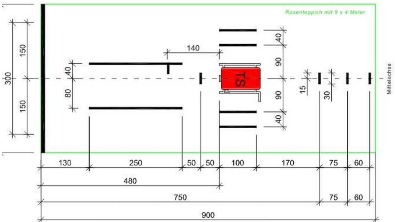
Abb.1: Bodenmarkierung für das Aufstellen der Wettbewerbsgeräte
