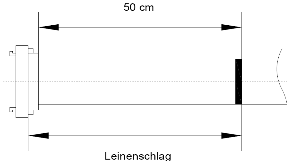
Abb.20: Anbringung der Markierung auf dem Saugschlauch und schematische Darstellung des Bereiches für den Leinenschlag
