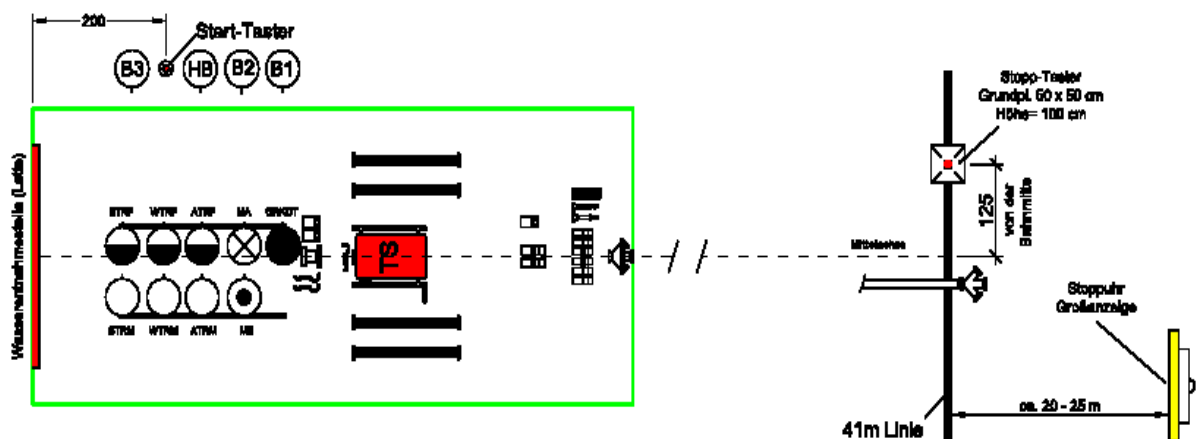
Abb.46: Aufbau der elektronischen Zeitnehmung
